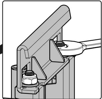
Arm Tension Nuts Écrous de tension du bras
